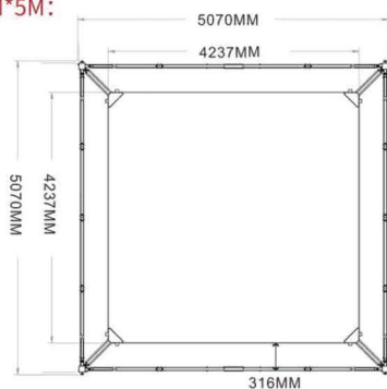
Dimensiones del ring desplegado
