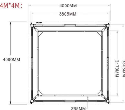
Dimensiones del ring desplegado
