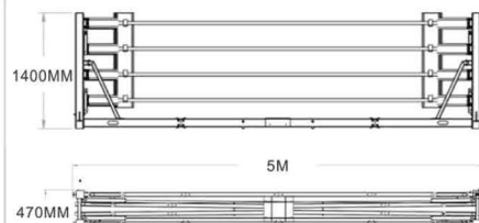
Dimensiones del ring plegado
